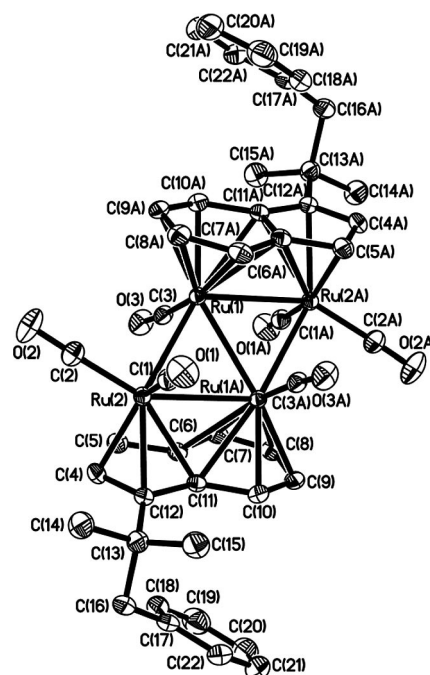
Figure 4. ORTEP diagram of 14 . Selected bond lengths [Å]: Ru(1)–Ru(1A) 2.7461(7), Ru(1)–Ru(2A) 2.8233(6), Ru(1)–Ru(2) 2.7287(5), Ru(1)–C(6A) 2.472(3), Ru(1)–C(7A) 2.370(4), Ru(1)–C(8A) 2.312(4), Ru(1)–C(9A) 2.245(3), Ru(1)–C(10A) 2.204(4), Ru(1)–C(11A) 2.408(3), Ru(2)–C(4) 2.205(4), Ru(2)–C(5) 2.314(4), Ru(2)–C(6) 2.562(3), Ru(2)–C(11) 2.499(3), Ru(2)–C(12) 2.269(4), C(6)–C(7) 1.408(5), C(6)–C(11) 1.455(5), C(7)–C(8) 1.398(5), C(8)–C(9) 1.394(5), C(9)–C(10) 1.412(5), C(10)–C(11) 1.436(5).
