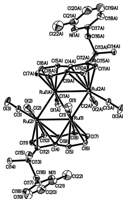
Figure 3. Molecular structure of 10 . Selected bond lengths [Å]: Ru(1)–Ru(1A) 2.7266(8), Ru(1)–Ru(2A) 2.7354(6), Ru(1)–Ru(2) 2.8223(6), Ru(1)–C(4) 2.419(5), Ru(1)–C(5) 2.224(5), Ru(1)–C(6) 2.234(5), Ru(1)–C(7) 2.296(5), Ru(1)–C(8) 2.367(5), Ru(1)–C(9) 2.464(5), Ru(2)–C(4) 2.499(4), Ru(2)–C(9) 2.573(4), Ru(2)–C(10) 2.319(5), Ru(2)–C(11) 2.210(5), Ru(2)–C(12) 2.282(5), C(4)–C(5) 1.431(6), C(4)–C(9) 1.450(6), C(5)–C(6) 1.421(7), C(6)–C(7) 1.398(7), C(7)–C(8) 1.407(7), C(8)–C(9) 1.415(6).
